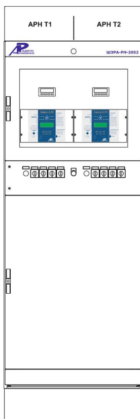
Шкаф регулирования напряжения трансформаторов ШЭРА-РН-2052 (БПВА.656457.137, БПВА.650645.001 ТУ)
